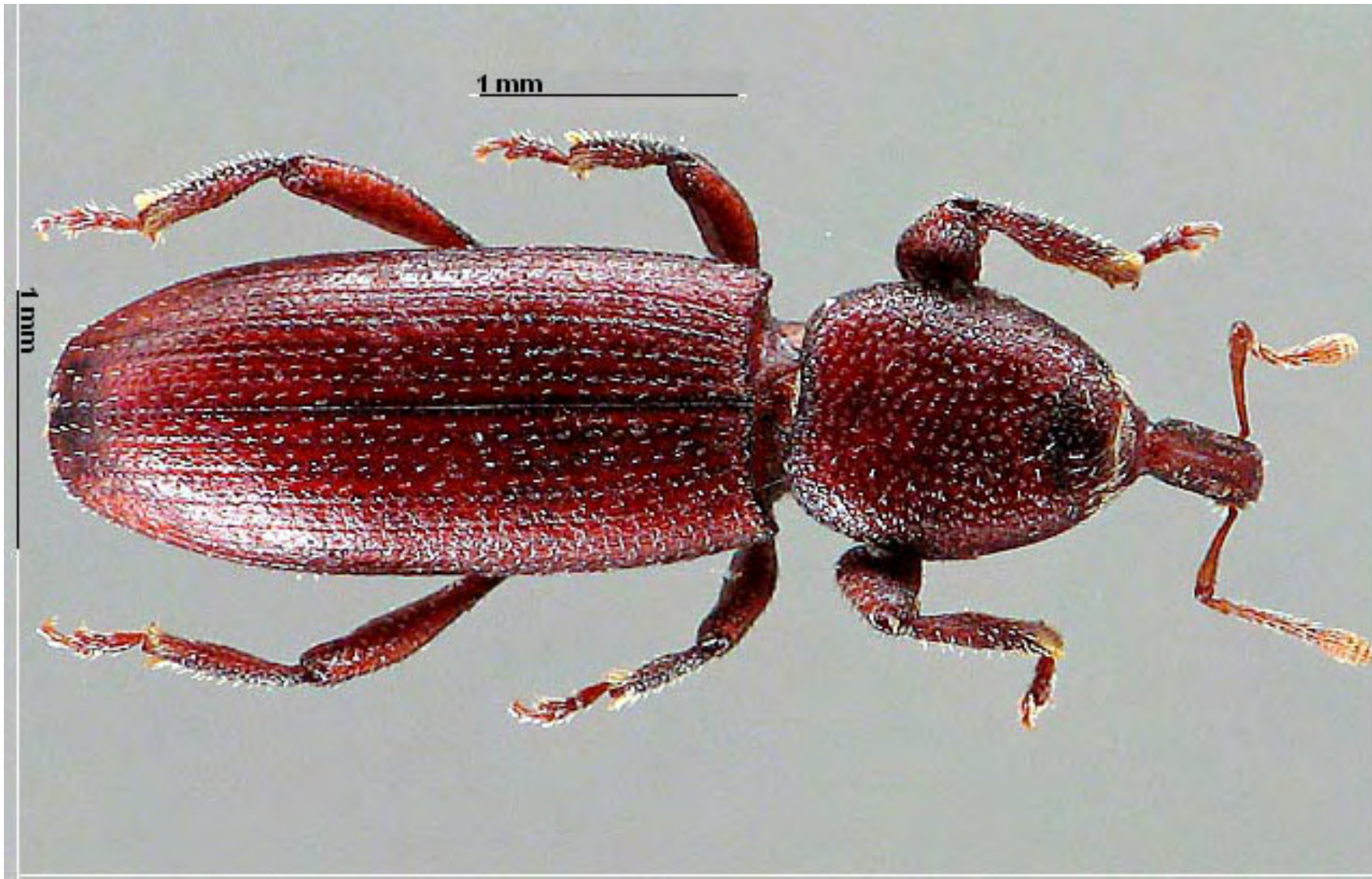
Torneuma troglodytis
